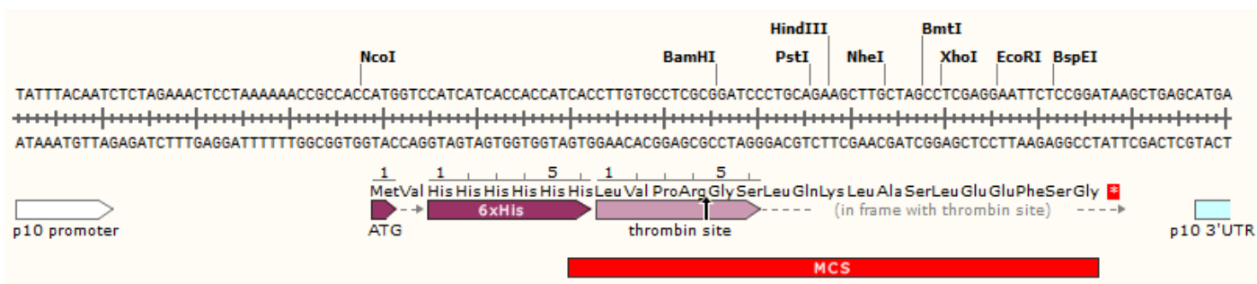
pQB4a 启动子/多克隆位点细节图
